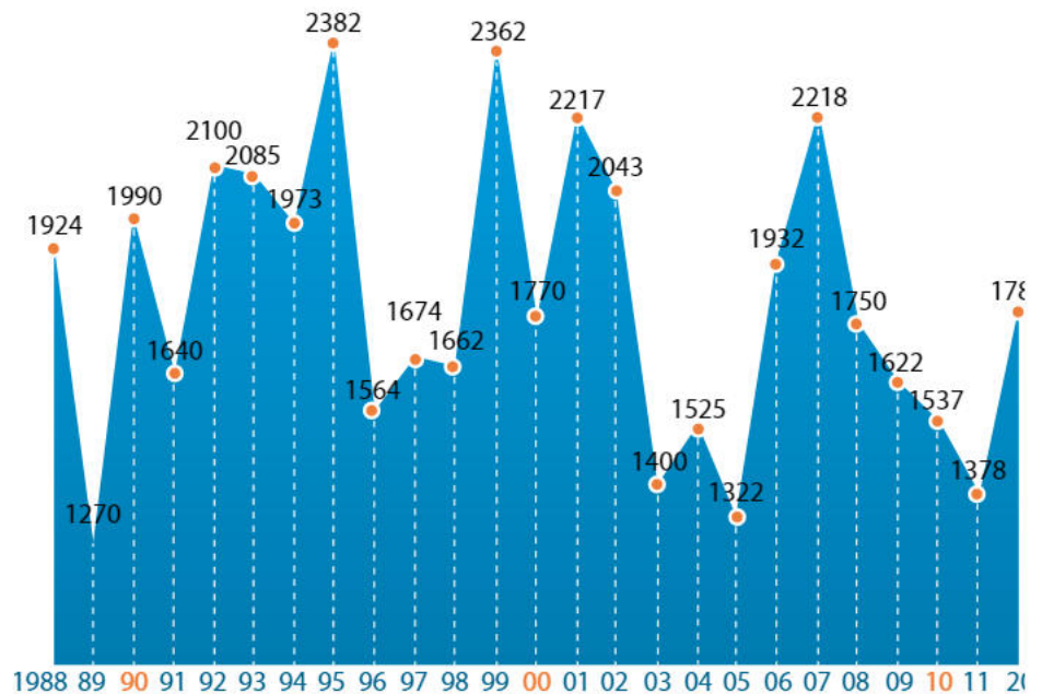
Précipitations annuelles sur les 25 dernières années (en mm)
