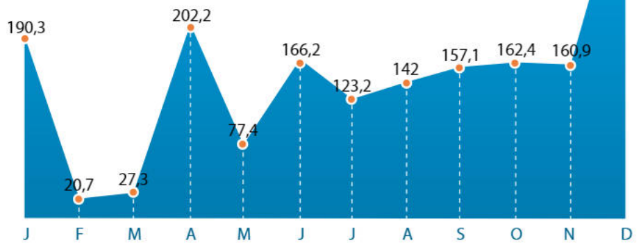
Précipitations de l'année 2012 (en mm)
